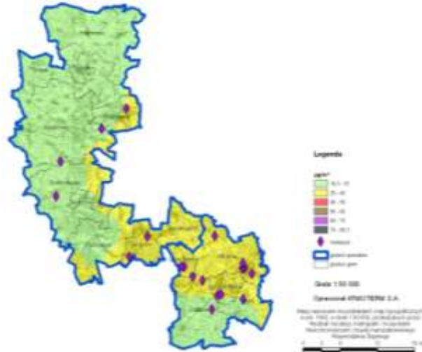
Strefa gliwicko-mikołowska - rozkład stężeń średniorocznych pyłu zaw. PM10 - rok bazowy 2009
